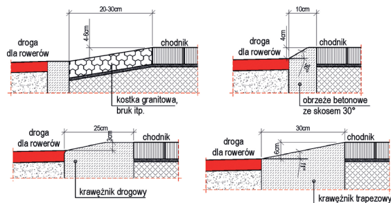
SCHEMAT 14. Przykładowe obniżenia drogi dla rowerów względem chodnika.
