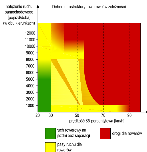
SCHEMAT 4. Orientacyjny stopień separacji ruchu rowerowego od samochodowego w zależności od natężenia ruchu samochodowego na drodze.
