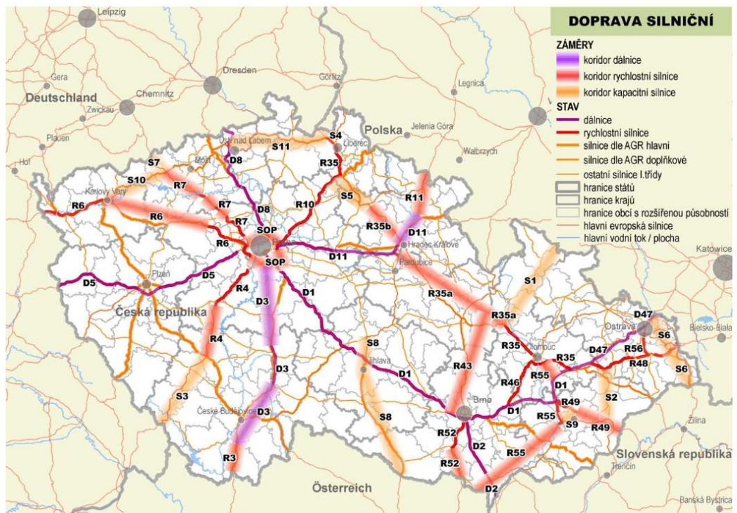
Rysunek 3 Kierunki rozwoju transportu drogowego zawarte w polityce rozwoju przestrzennego Republiki Czeskiej z 2008 r.
